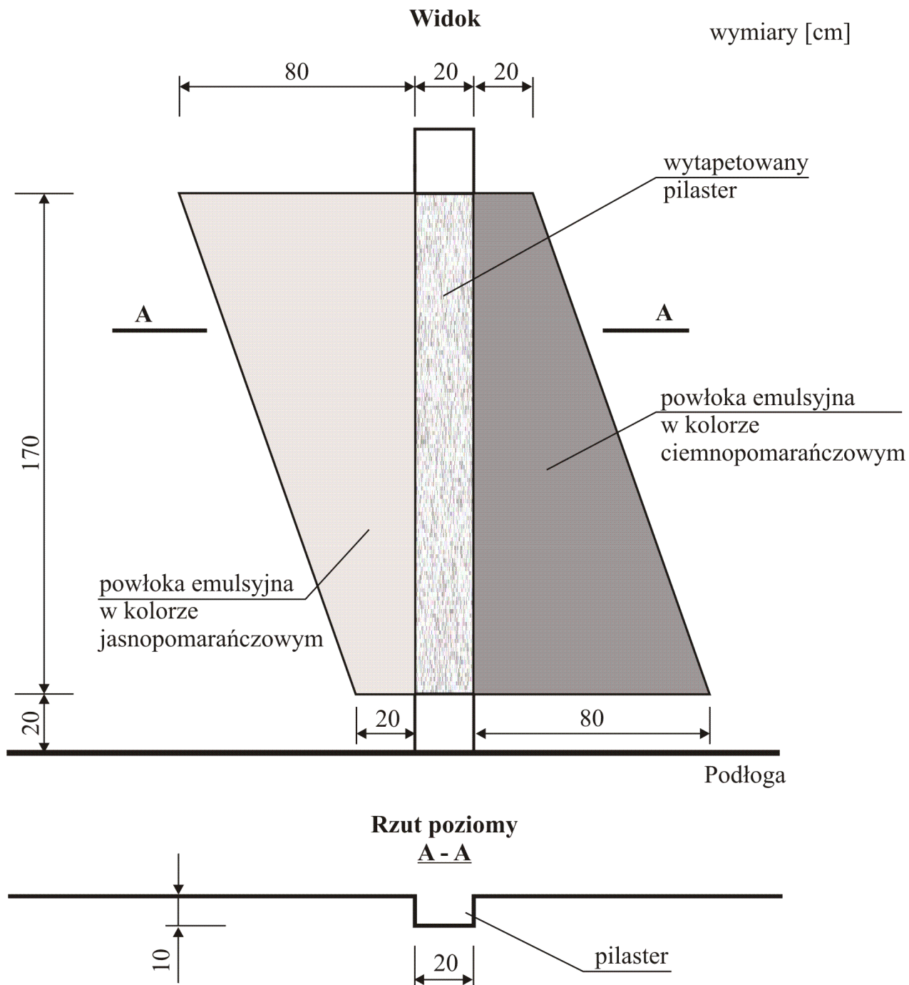
Rys. Widok i rzut poziomy ściany z pilastrem
