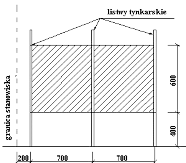
Rysunek 2. Widok ściany przeznaczonej do wykonania narzutu
