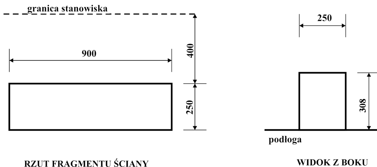
Rysunek 1. Widok fragmentu ściany do wymurowania
