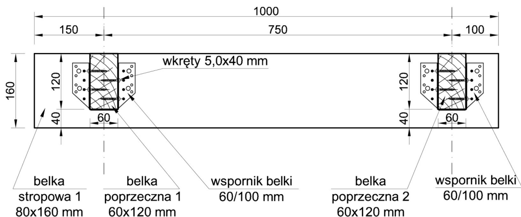
Rysunek 2. Przekrój A-A fragmentu stropu drewnianego
