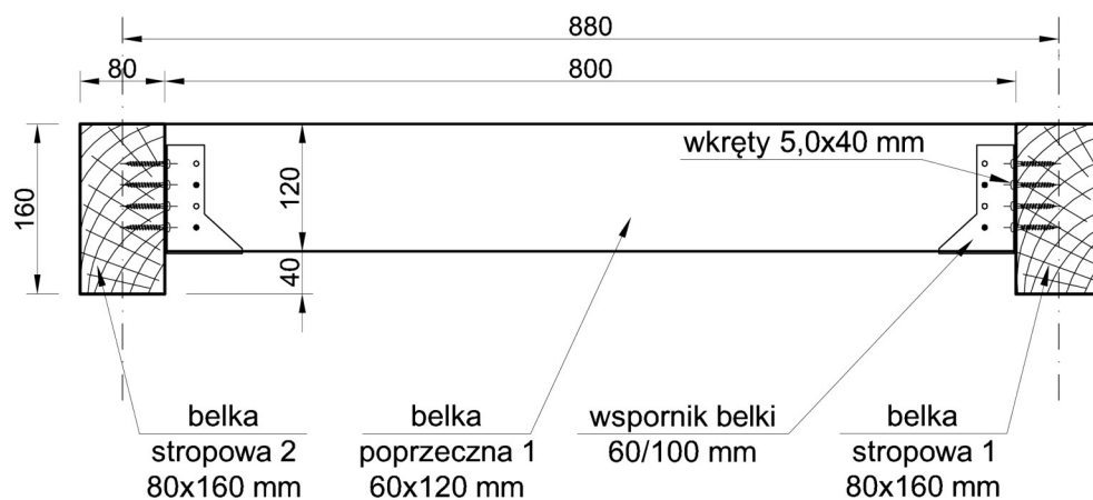
Rysunek 3. Przekrój B-B fragmentu stropu drewnianego
