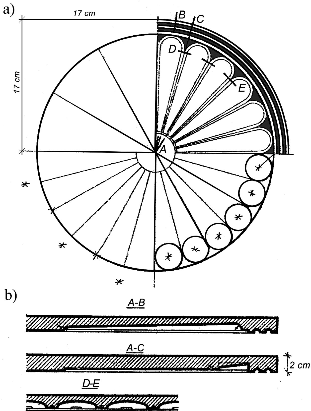
Rysunek 2. Rysowanie rozety o układzie promienistym: a) kolejność rysowania, b) przekroje modelu sztukatorskiego
