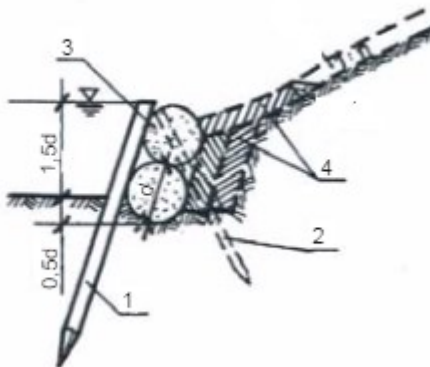
Rysunek. Umocnienie podstawy skarpy podwójną kiską faszynową 1 – kołek faszynowy, 2 – szpilka, 3 – kieszka faszynowa, 4 – darnina
