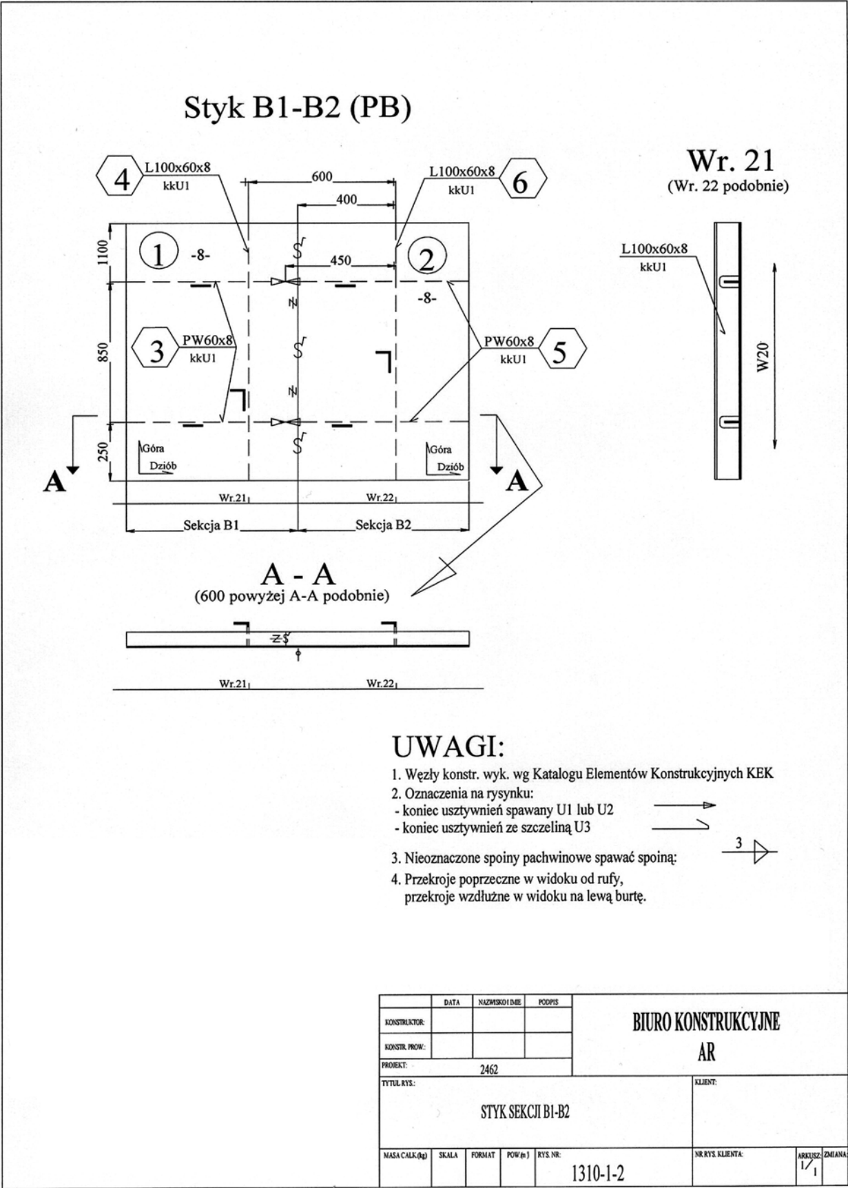
Rysunek 1. Styk B1-B2 (PB)
