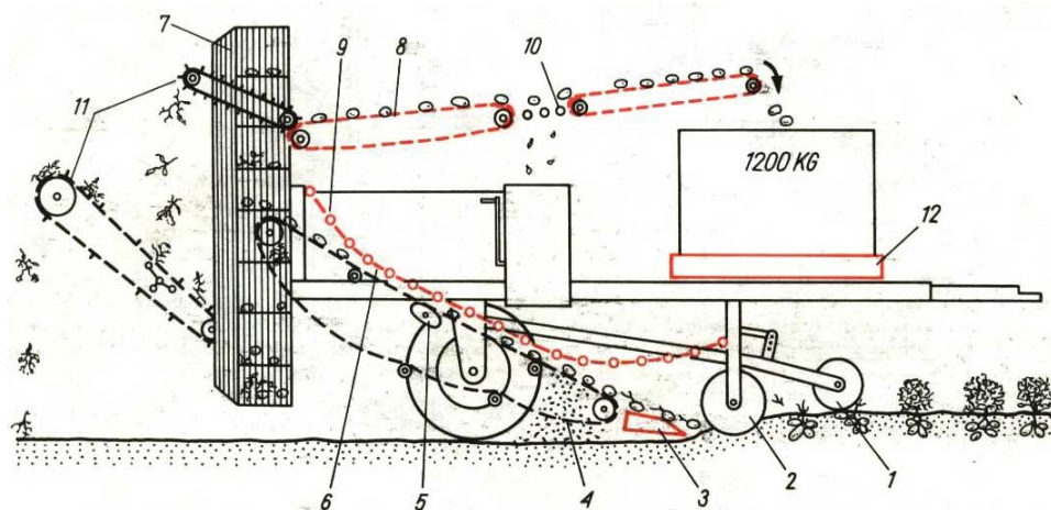
Rys. 6/XIV. Kombajn jednorzędowy do zbioru ziemniaków Z-644 Anna: 1 - rolka kopiująca, 2 - krój tarczowy, 3 - lemiesz płytkowy, 4 - przenośnik odsiewający, 5 - wstrząsacz eliptyczny, 6 - drabinka krusząca bryły, 7 - bęben obrotowy, 8 - stół selekcyjny, 9 - pomost obsługi stołu, 10 - odsiewacz drobnych zanieczyszczeń, 11 - oddzielacz lętwów, 12 - przenośnik podłogowy
